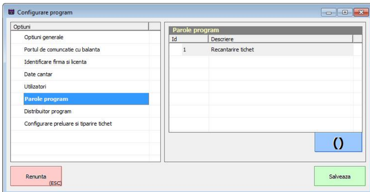
Fig. 14: parolele programului
